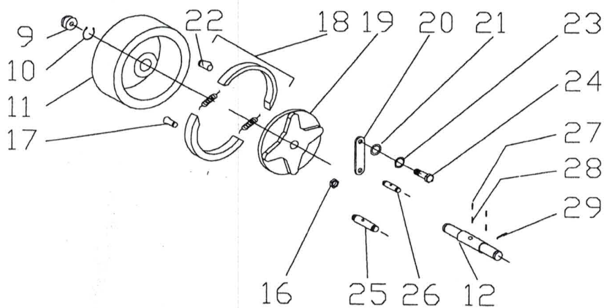
Lenkrad mit Bremse
