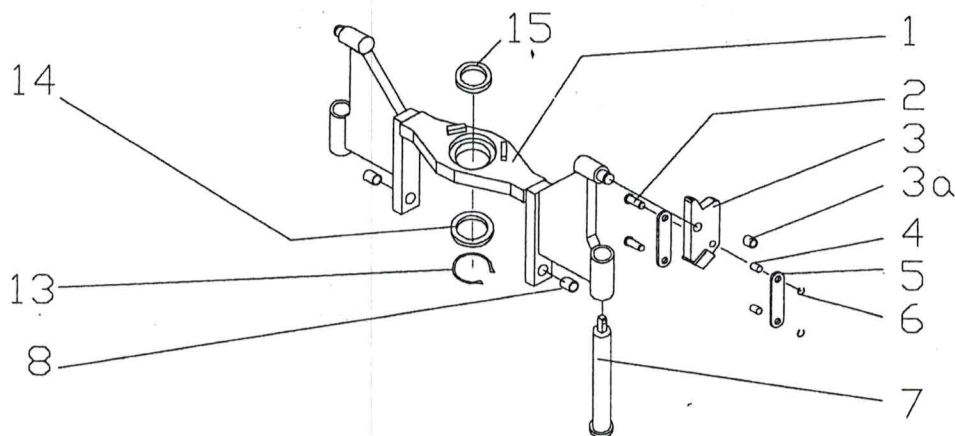
Lenkrad ohne Bremse
